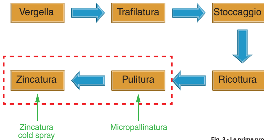
Fig. 2 - Il progetto Ultra Crash Treatment si pone l'obiettivo di affrontare un problema ambientale collegato al processo di produzione del filo trafileato zincato, intervenendo in due determinate fasi del ciclo produttivo, quella di pulitura del filo cotto e quella di zincatura vero e proprio, evidenziato nel diagramma di flusso produttivo qui riportato
