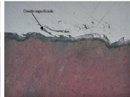
Fig. 3 - Le prime prove effettuate con graniglia metallica hanno mostrato da un lato la rimozione degli ossidi formati sul filo cotto, dall'altro la formazione di danni superficiali tali da ridurre la resistenza del filo o da provocare ripercussioni negative sulla successiva fase di zincatura
