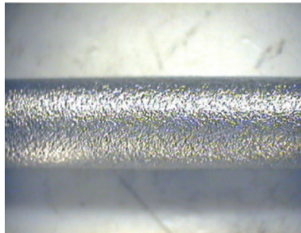
Fig. 3 - Le prime prove effettuate con graniglia metallica hanno mostrato da un lato la rimozione degli ossidi formati sul filo cotto, dall'altro la formazione di danni superficiali tali da ridurre la resistenza del filo o da provocare ripercussioni negative sulla successiva fase di zincatura
