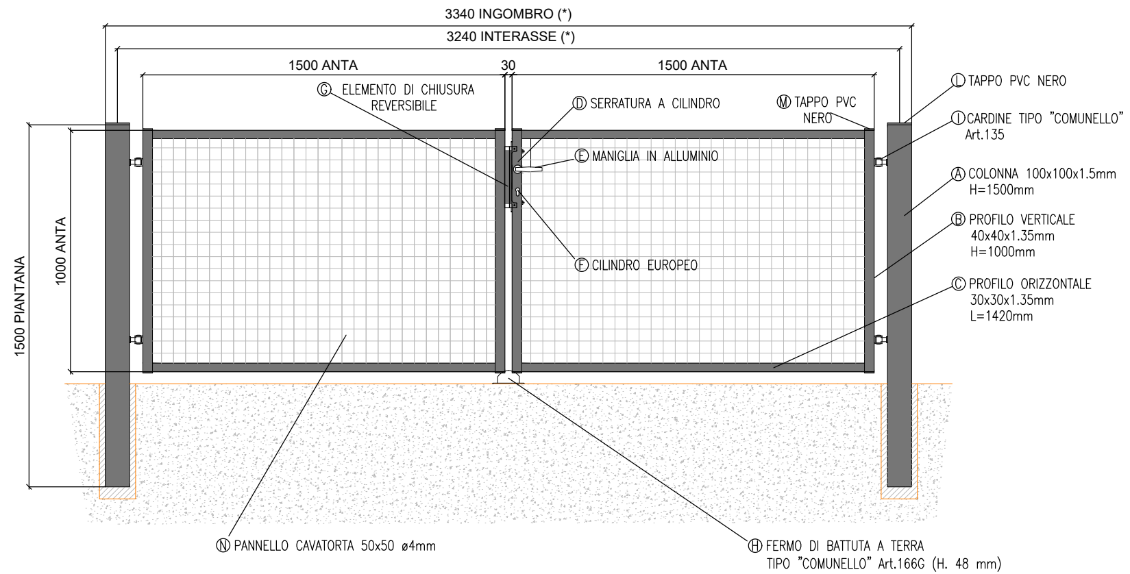
FIG. 1: DETTAGLIO ANTA-COLONNA
