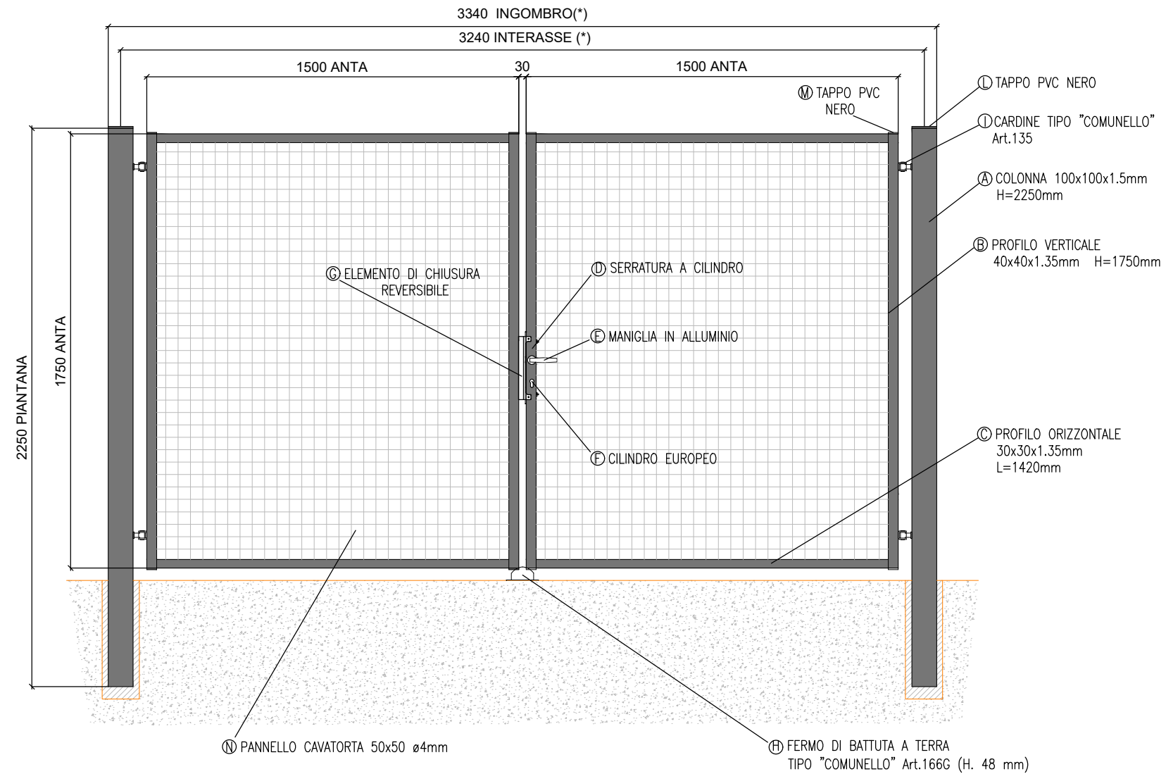
FIG. 1: DETTAGLIO ANTA-COLONNA
