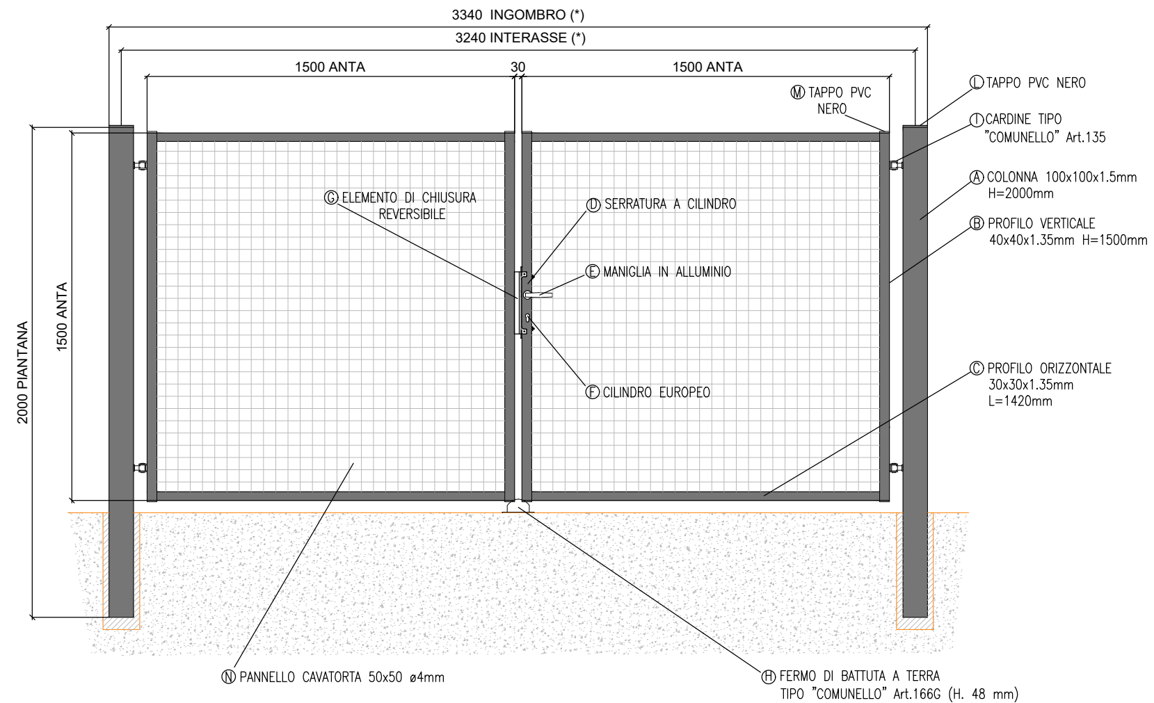
FIG. 1: DETTAGLIO ANTA-COLONNA
