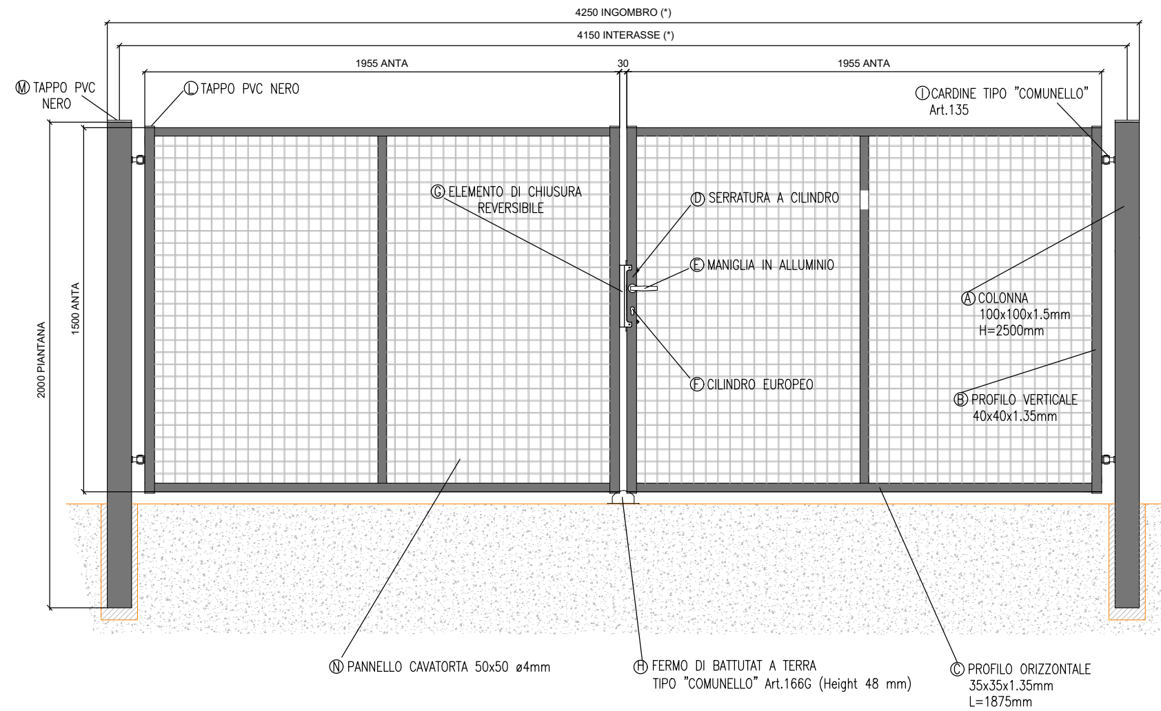
FIG. 1: DETTAGLIO ANTA-COLONNA
