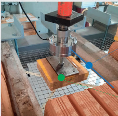
Test con carico concentrato applicato con martinetto (prova su 1 punto di carico)
