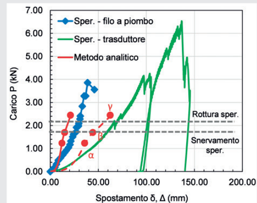
Test con carico uniformemente distribuito applicato con sacchi di sabbia
