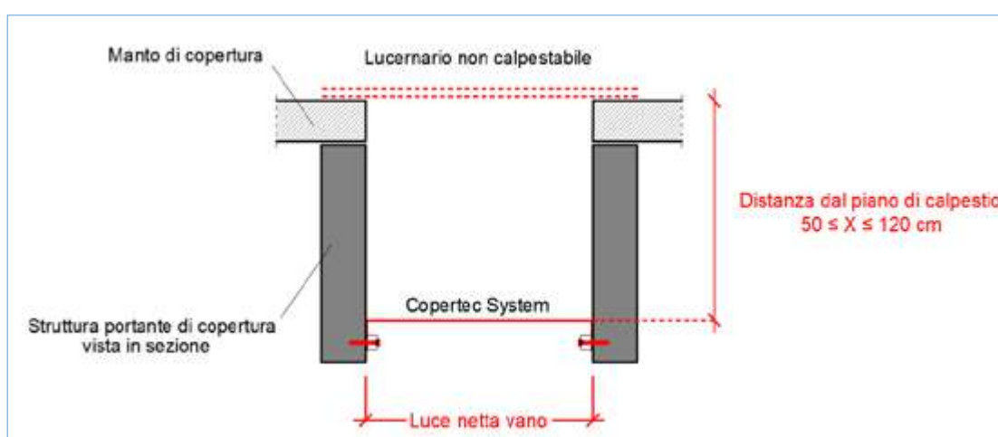
Fig. 20 – Schema con posizionamento reti lontane da piano di calpestio (Schemi di posa A, B e C).
