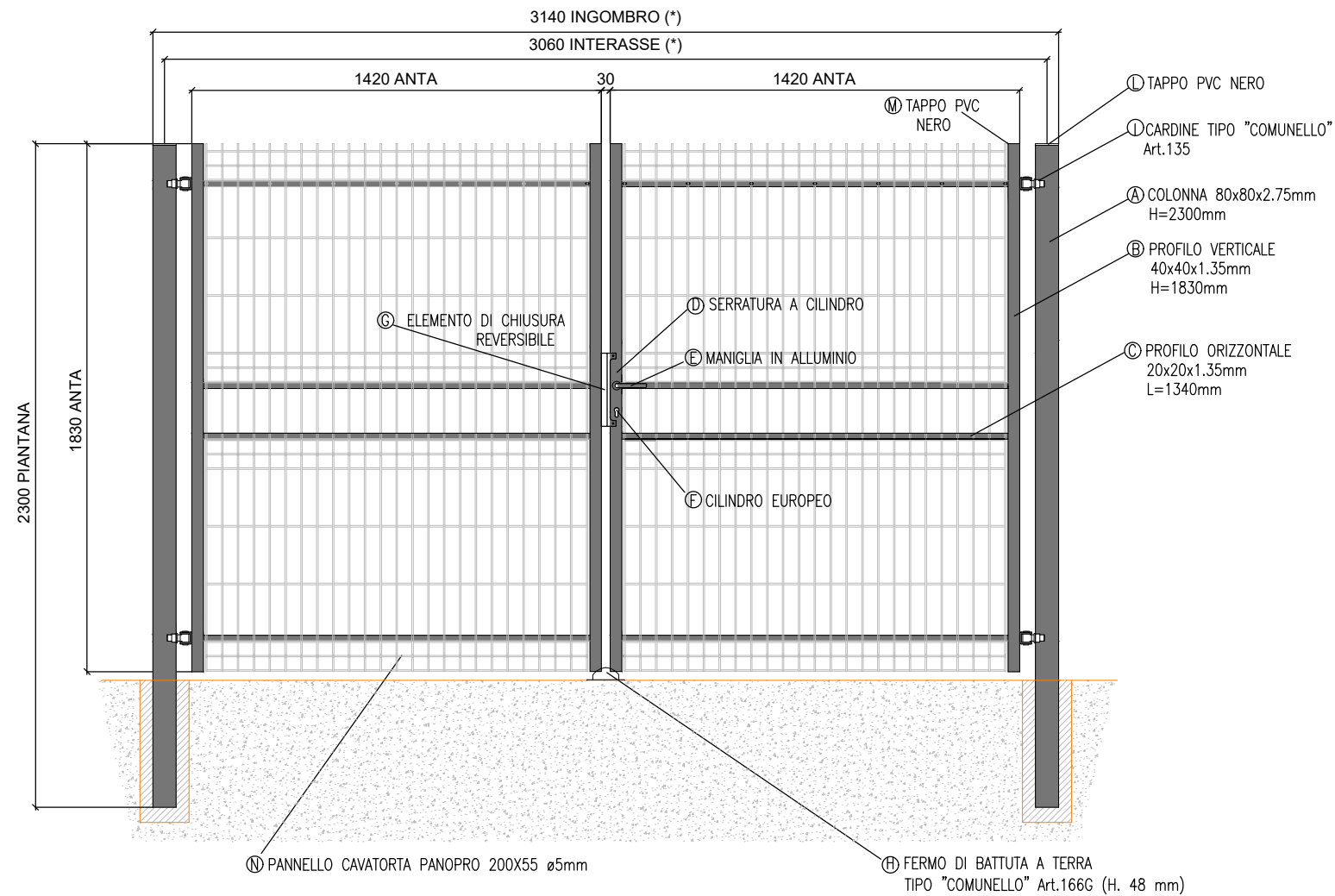
FIG. 1: DETTAGLIO ANTA-COLONNA
