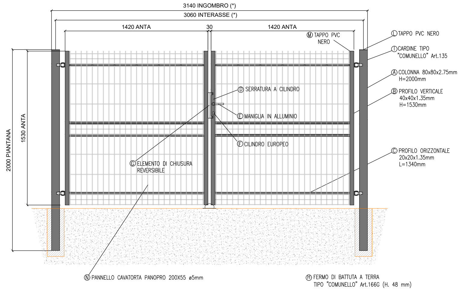
FIG. 1: DETTAGLIO ANTA-COLONNA
