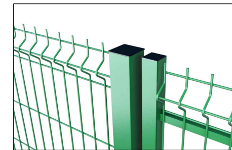
FIG. 1: DETTAGLIO ANTA-COLONNA
